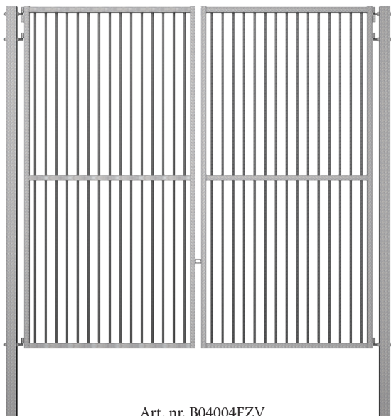
Art. nr. B04004FZV DG 4000x4000 FZV
