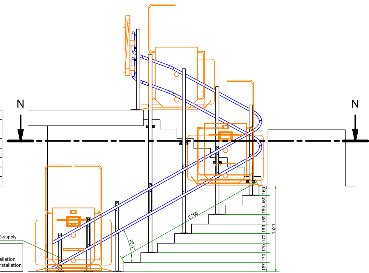
N-N ( 1 : 40 )
