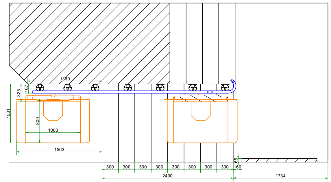
N-N ( 1 : 40 )
