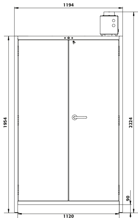
Framprofil
